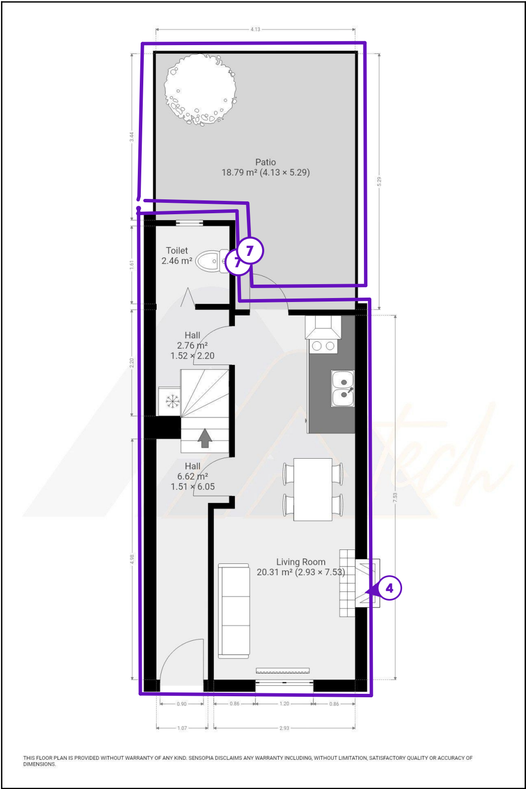
Legende van plan 1.4: grondplan GLVL niv +0 algemeen
