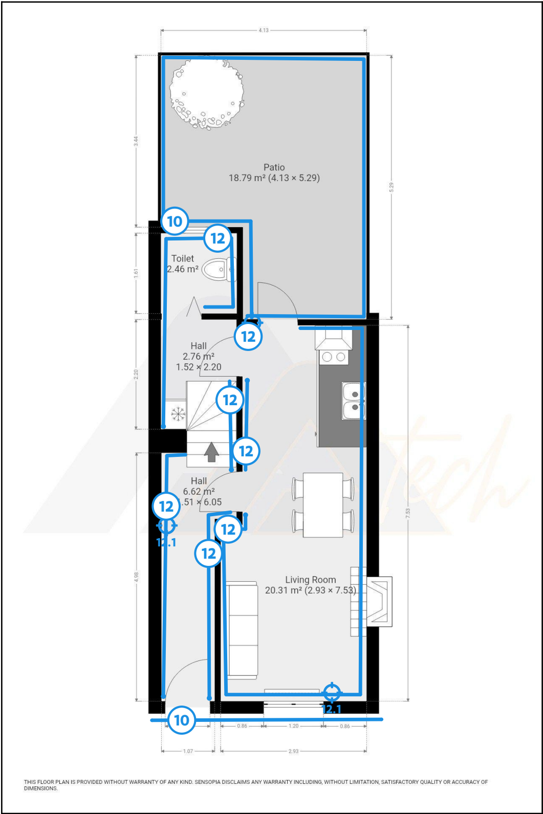
Legende van plan 1.2: grondplan GLVL niv +0 muren
