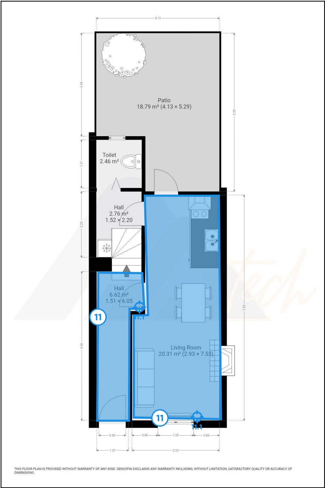
Legende van plan 1.3: grondplan GLVL niv +0 plafonds
